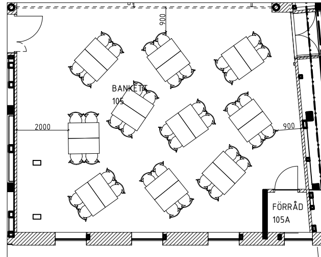
3 MÖBEL-LAYOUT 3 SCALE: 1:150 ANTAL PLATSER: 40 PLATSER
