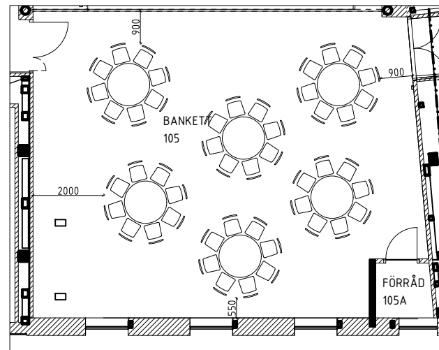
6 MÖBEL-LAYOUT 6 SCALE: 1:150 ANTAL PLATSER: 48 PLATSER
