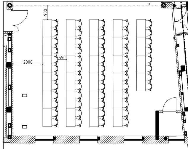
1 MÖBEL-LAYOUT 1 SCALE: 1:150 ANTAL PLATSER: 56 PLATSER
