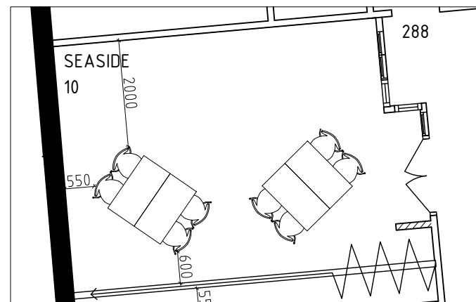
4 MÖBEL-LAYOUT 4 SCALE: 1:100 ANTAL PLATSER: 8 PLATSER
