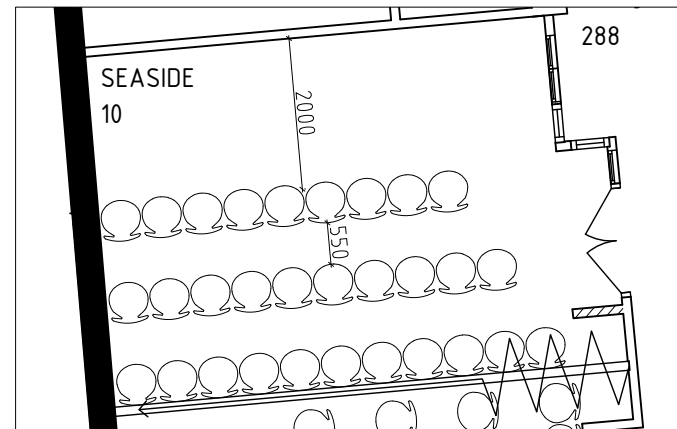
2 MÖBEL-LAYOUT 2 SCALE: 1:100 ANTAL PLATSER: 30 PLATSER
