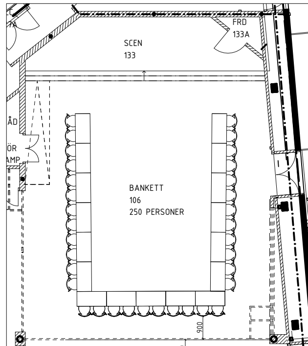
5 MÖBEL-LAYOUT 5 SCALE: 1:150
