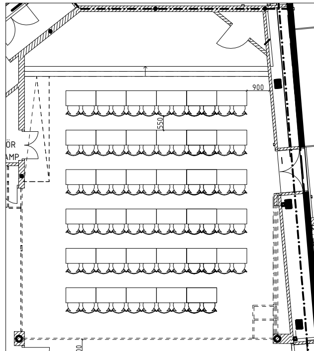
1 MÖBEL-LAYOUT 1 SCALE: 1:150
