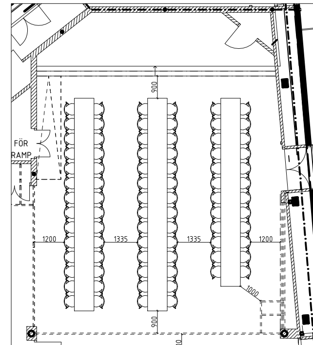
7 MÖBEL-LAYOUT 7 SCALE: 1:150
