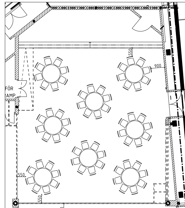
6 MÖBEL-LAYOUT 6 SCALE: 1:150
