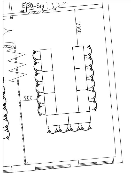
4 MÖBEL-LAYOUT 4 SCALE: 1:100 ANTAL PLATSER: 16 PLATSER
