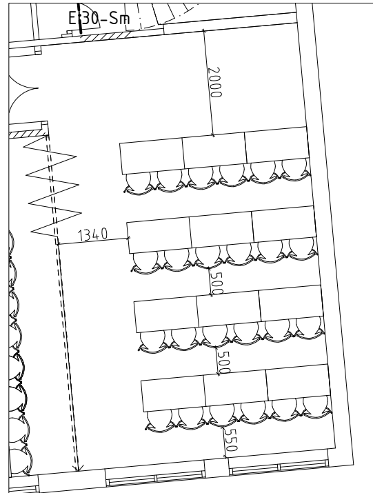
1 MÖBEL-LAYOUT 1 SCALE: 1:100 ANTAL PLATSER: 24 PLATSER
