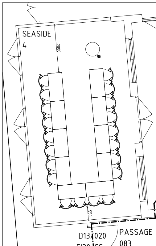
3 MÖBEL-LAYOUT 3 SCALE: 1:100
