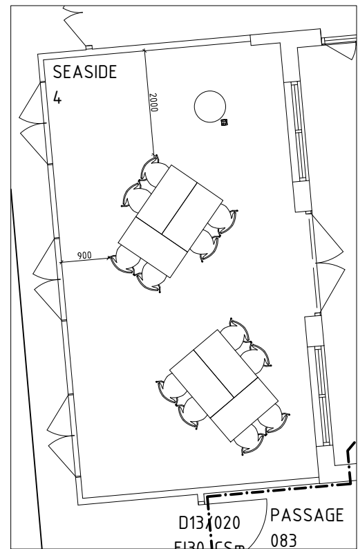
5 MÖBEL-LAYOUT 5 SCALE: 1:100
