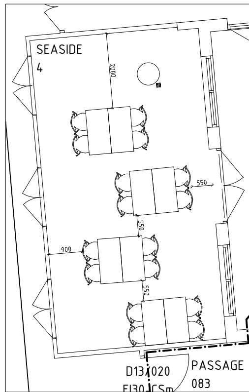
4 MÖBEL-LAYOUT 4 SCALE: 1:100
