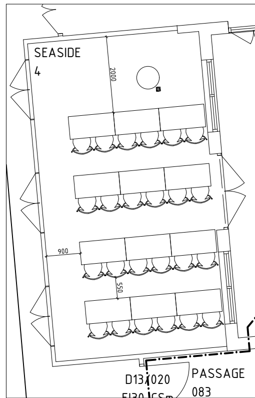
2 MÖBEL-LAYOUT 2 SCALE: 1:100
