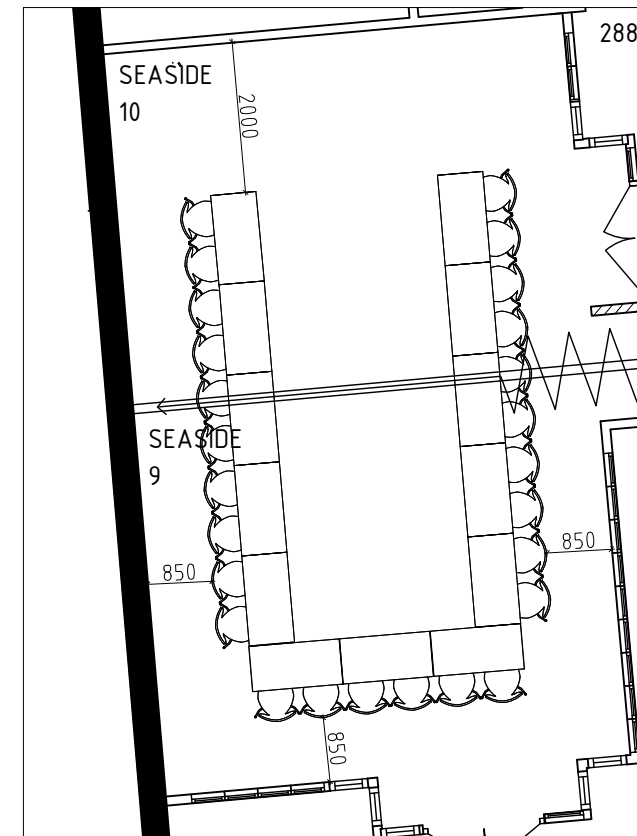
3 MÖBEL-LAYOUT 3 SCALE: 1:100 ANTAL PLATSER: 26 PLATSER
