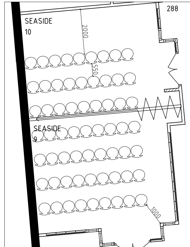
1 MÖBEL-LAYOUT 1 SCALE: 1:100 ANTAL PLATSER: 63 PLATSER
