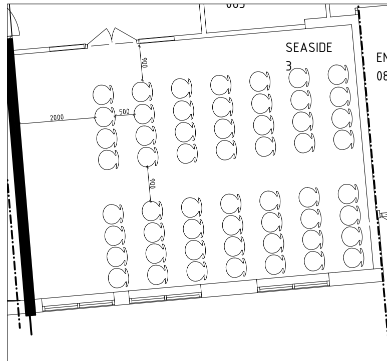
1 MÖBEL-LAYOUT 1 SCALE: 1:100
