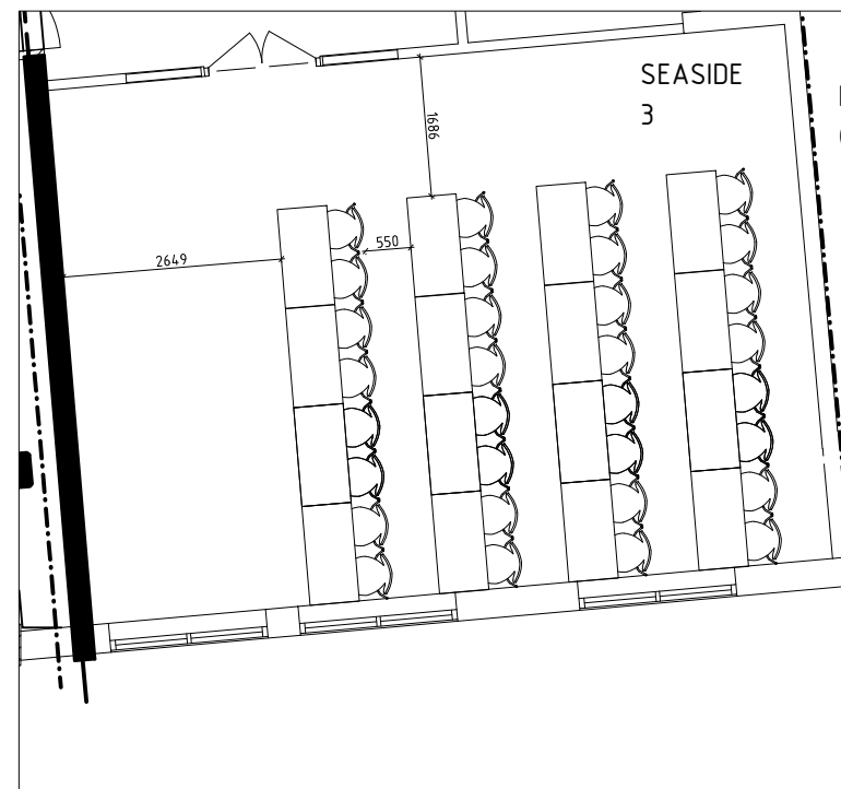
2 MÖBEL-LAYOUT 2 SCALE: 1:100
